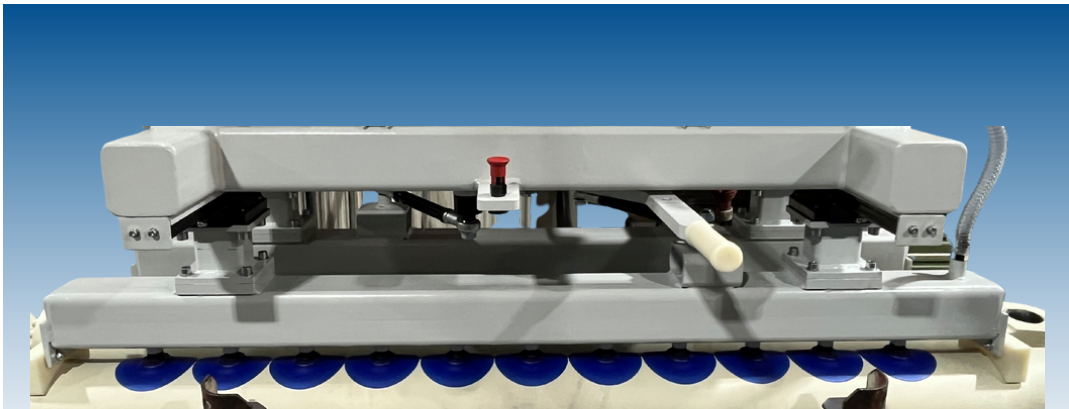
Saugtraverse Seitenansicht
