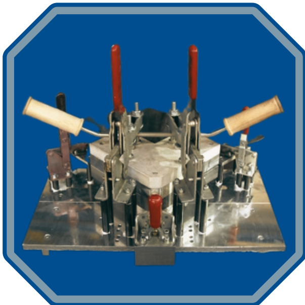
Eckschweißmaschine
